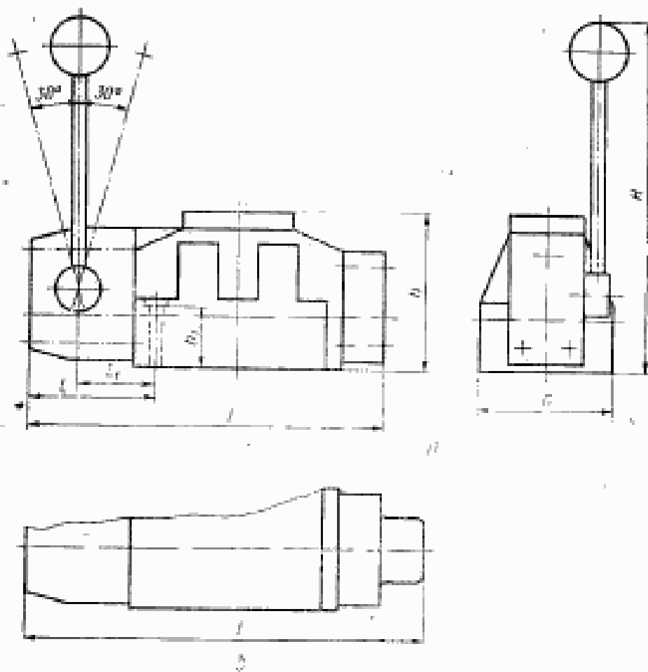
а — трехпозиционный; б — двухпозиционный
