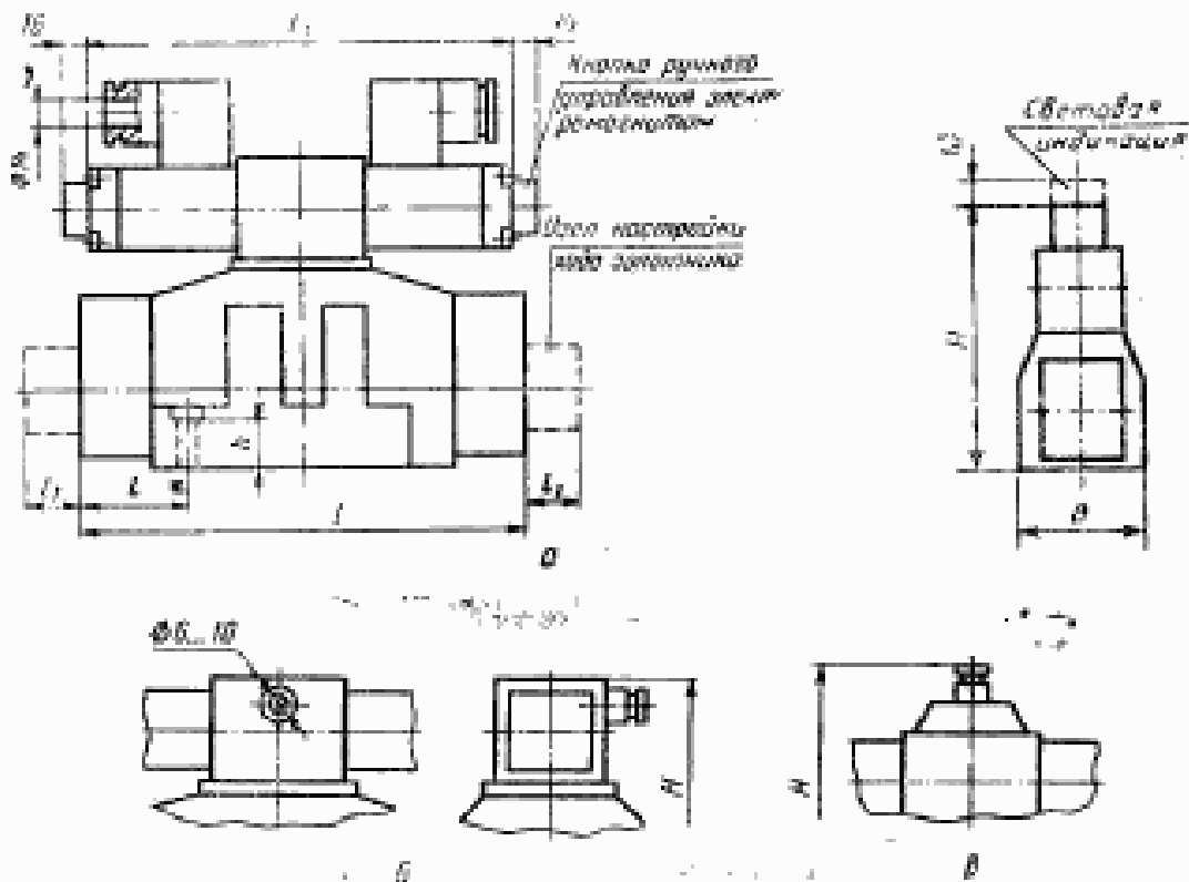
а — с подводом электрического кабеля через штепсельные разъемы; б — с подводом электрического кабеля сбоку; в — с подводом электрического кабеля сверху.
