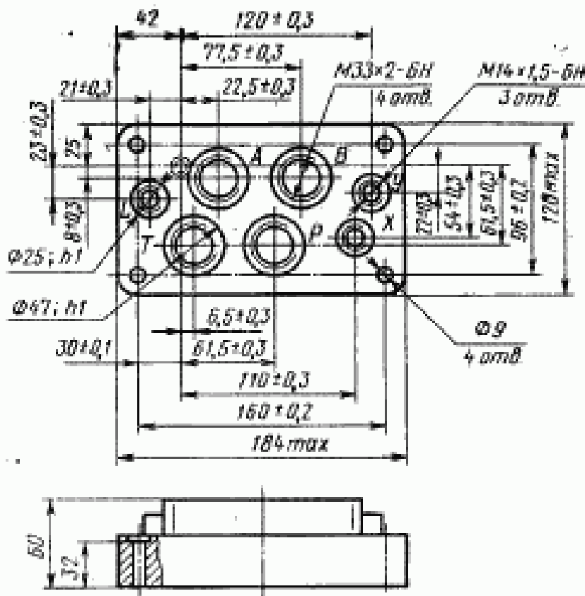
Масса 7,6 кг Черт. 3
